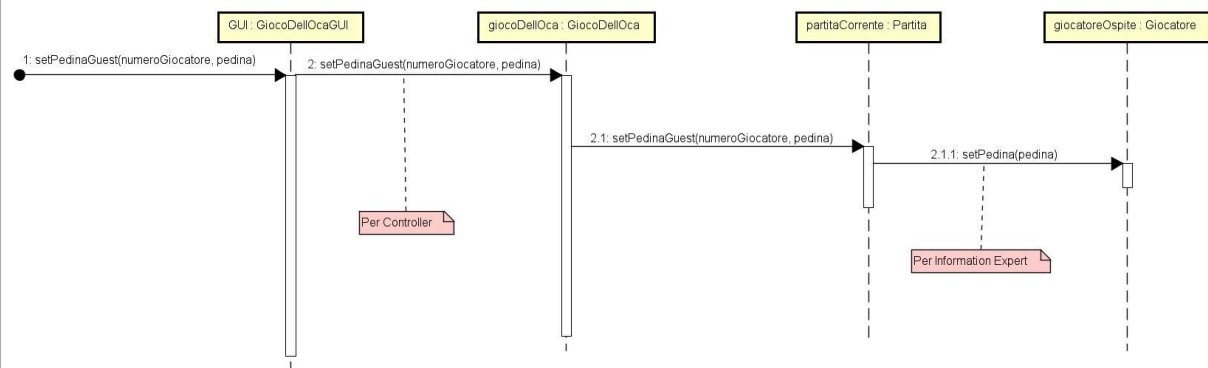
sd 13. UC4 SD setPedina (Giocatori ospiti)
