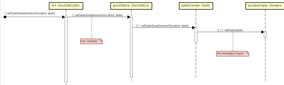
sd 12. UC4 SD setDado (Giocatori ospiti)
